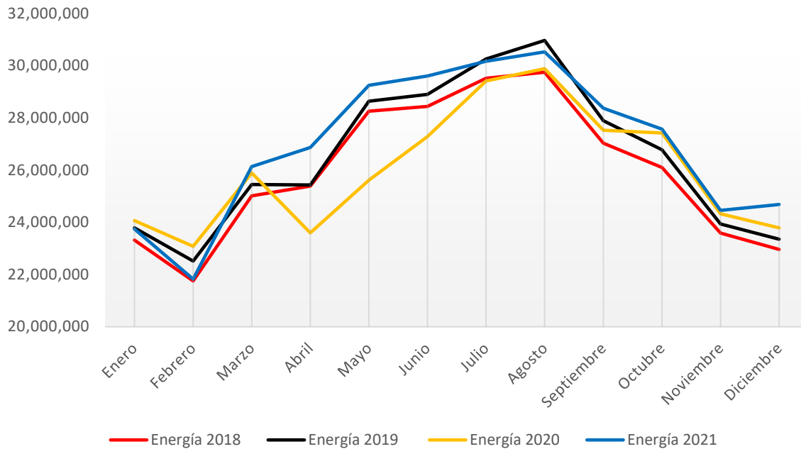
Gráfica 7. Volumen de Energía Eléctrica recibida en la Red Nacional de Transmisión (RNT) (MWh)
