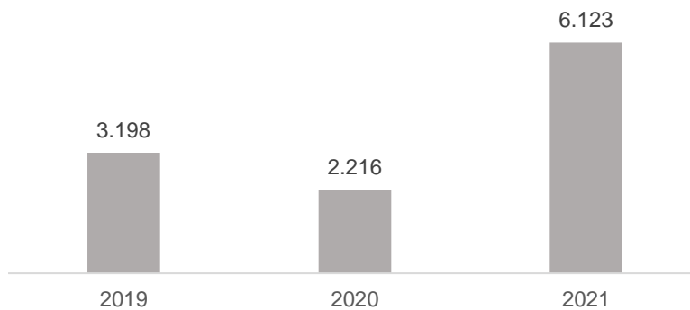
Gráfica 4. Índice Promedio de Duración de Interrupciones del Sistema (SAIDI) (Minutos)
