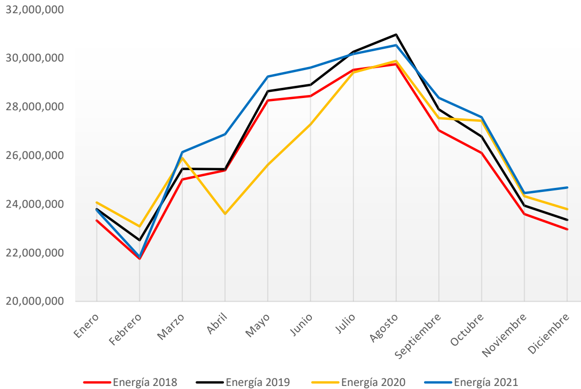
Gráfica 9. Volumen de Energía Eléctrica recibida en la Red Nacional de Transmisión 1 (MWh 2 )
