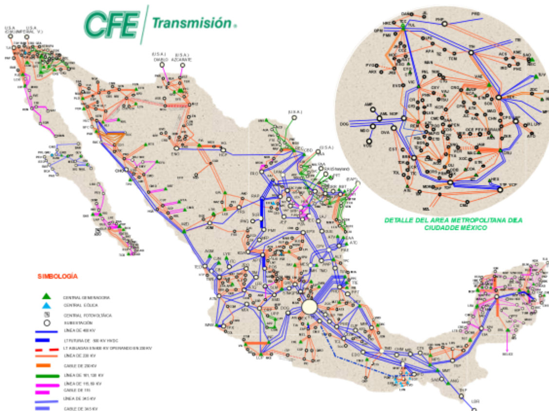
Ilustración 3. Red troncal de transmisión 2020
