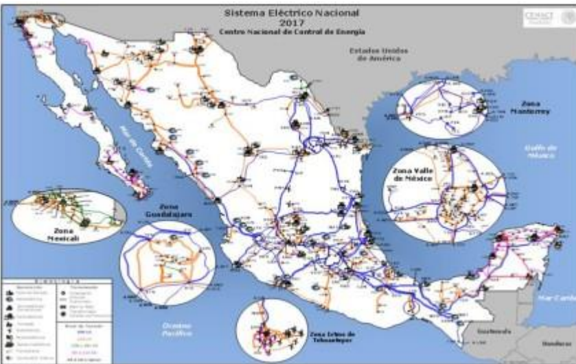
Gráfica 2. Red troncal de transmisión del SEN 2017
