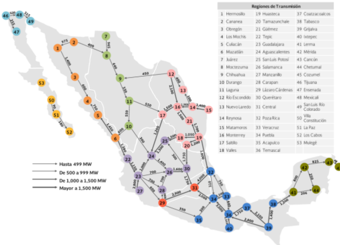
Ilustración 1. Capacidad de enlaces entre las 53 regiones de transmisión del SEN 2017
