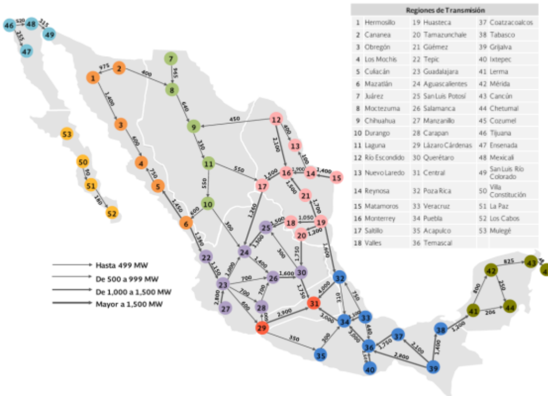
Ilustración 1. Capacidad de enlaces entre las 53 regiones de transmisión del SEN 2017
