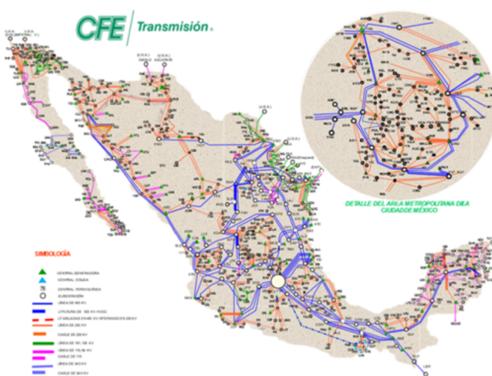
Ilustración 4. Red troncal de transmisión 2020
