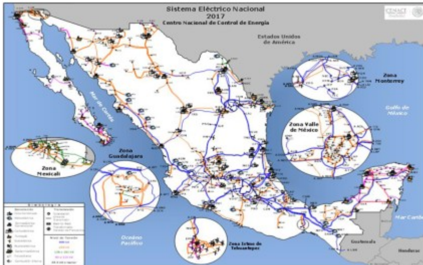
Gráfica 2. Red troncal de transmisión del SEN 2017
